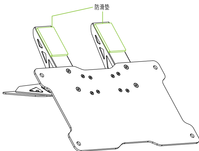
图5：可翻转踏板底板粘贴防滑垫，油门踏板和制动踏板各粘贴一片，即可完成组装。
