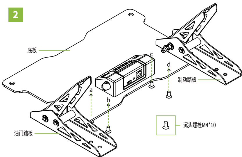
图2：将踏板放置于底板上，突出的转轴对准底板盒子的开口并推入开口内，用M4*10的沉头螺栓从底部向上锁紧，孔位以A-a，B-b，C-c，D-d的顺序对齐即可锁紧；
