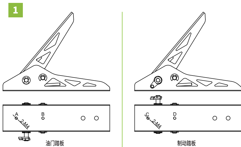
图1：取出制动踏板及油门踏板，校对安装孔位；
