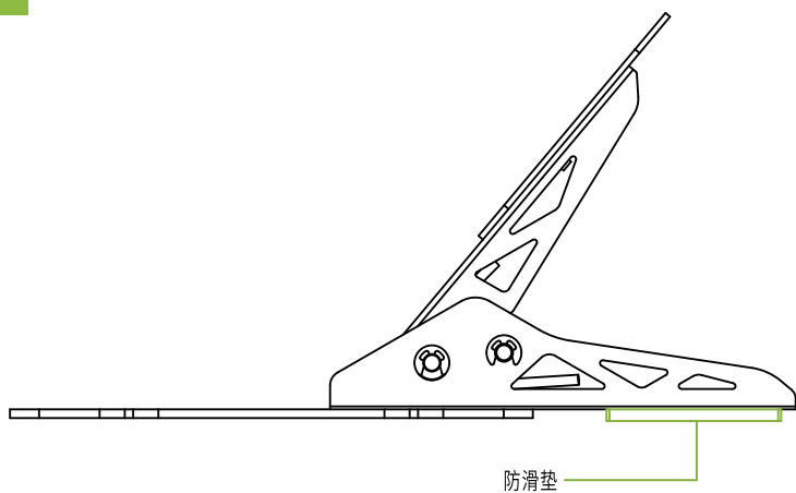
图4：取出防滑贴，撕掉贴膜后贴在踏板与底板未重合的悬空位置；
