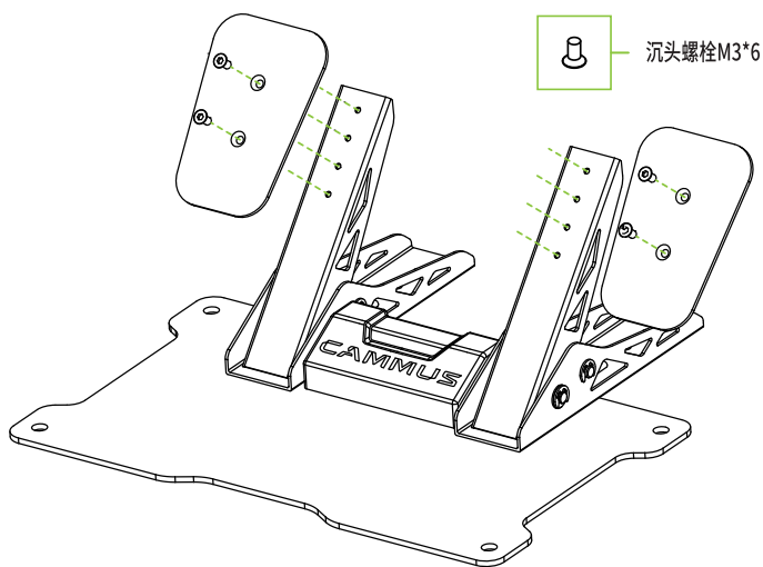
图3：踏板面的安装可根据个人需求选择安装孔位，取4颗M3*6的沉头螺栓对齐锁紧即可；
